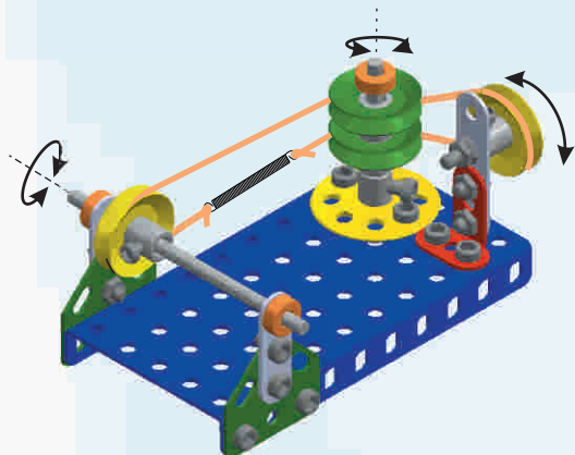
USA Example of free wheel gearing CZ Ukázka převodu přes volná kola D Beispiel des Losradgetriebes F Exemple de l'engrenage à roue mobile E Ejemplo del engranaje de ruedas locas NL Voorbeeld van transmissie via los rad H Furatoskerék-hajtómi példa I Esempio dell'ingranaggio a ruota folle SK Ukázka převodu cez voľné kolesá PL Przykład przełożenia przez wolne koło
