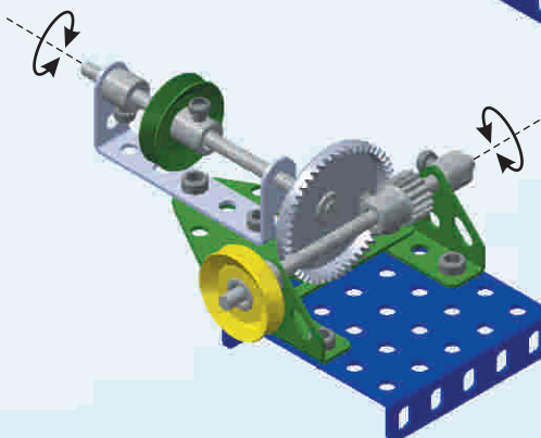
USA Example of free wheel gearing CZ Ukázka převodu přes volná kola D Beispiel des Losradgetriebes F Exemple de l'engrenage à roue mobile E Ejemplo del engranaje de ruedas locas NL Voorbeeld van transmissie via los rad H Furatoskerék-hajtómi példa I Esempio dell'ingranaggio a ruota folle SK Ukázka převodu cez voľné kolesá PL Przykład przełożenia przez wolne koło
